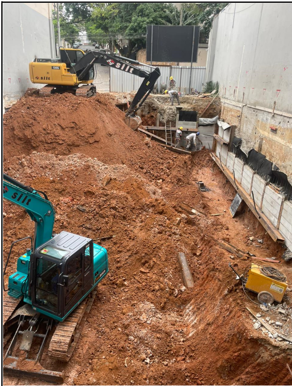
Escavação para execução dos serviços na entrada Santo Irineu.
